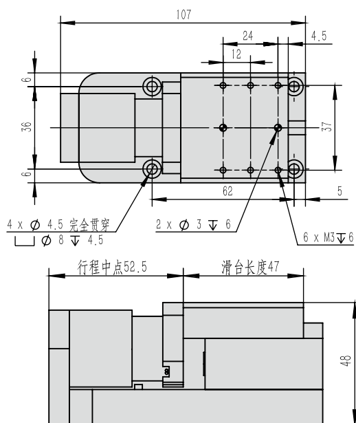
● 外形圖(單位:mm)
