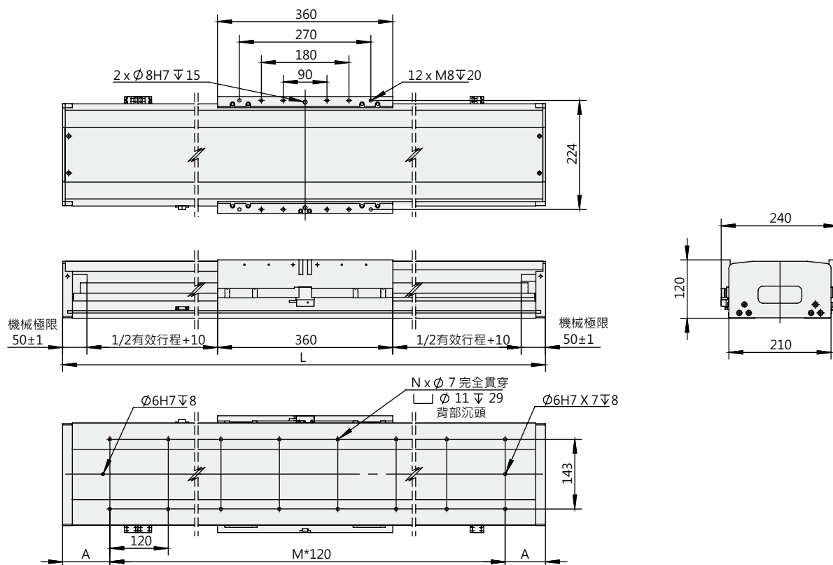
模組尺寸
